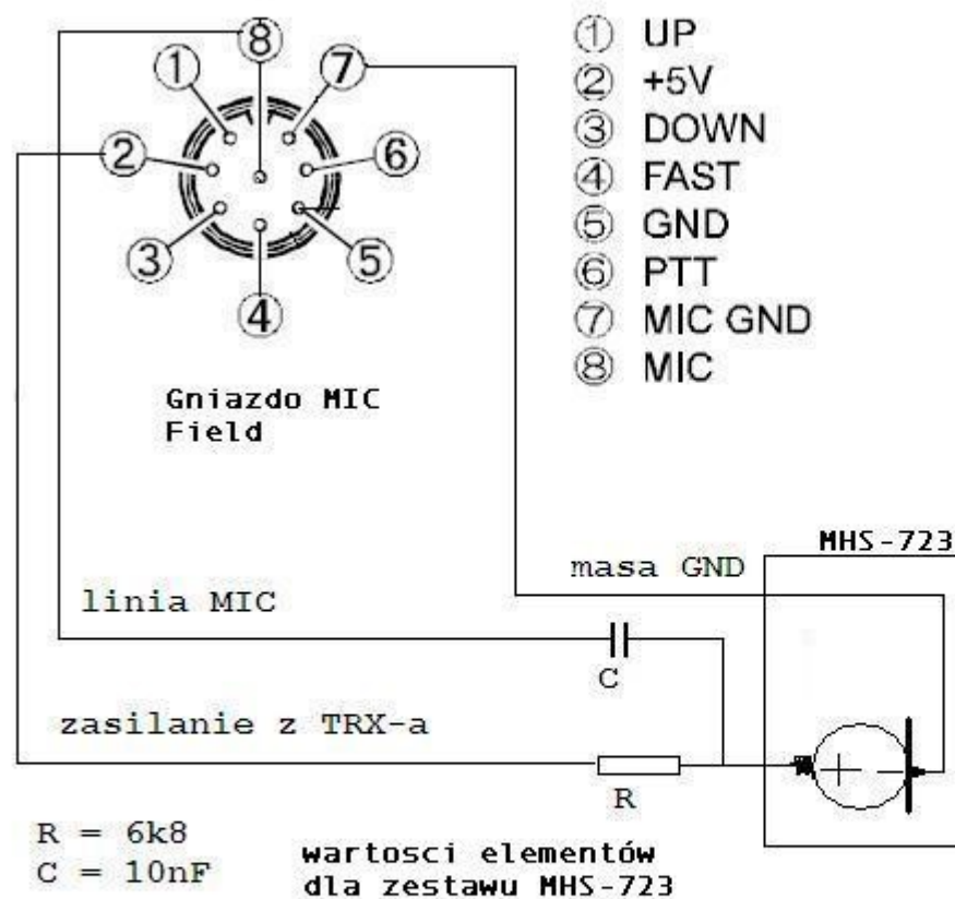
Schemat podłączenia mikrofonu elektr. do FT1000MP Field
